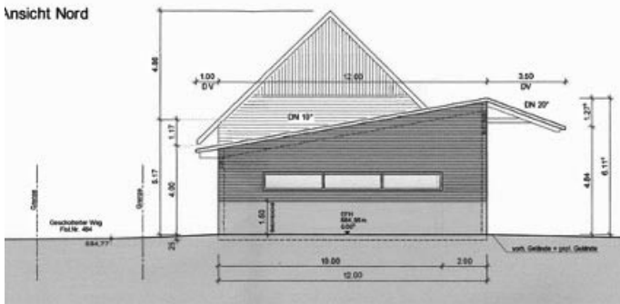
Ansicht Nord
